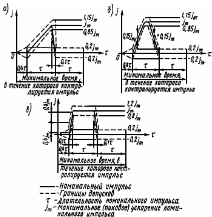
а - пилообразная, б - полусинусоидальная, в - трапецидальная.
