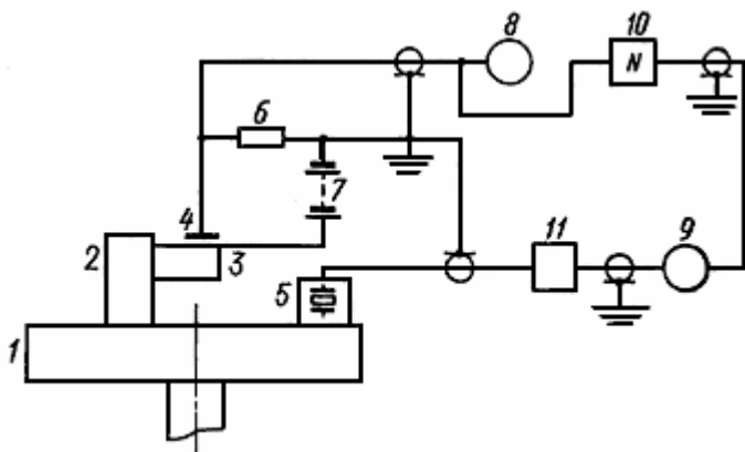
Принципиальная электрическая схема определения резонансных частот емкостным методом
