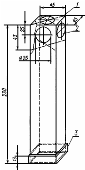
1 - направляющие перегородки; 2 - входные отверстия; 3 - съемное дно
